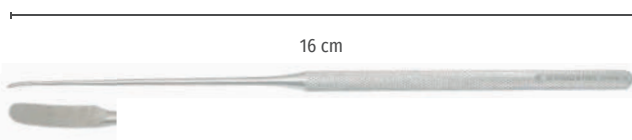
Beales Elevatorium, 1,5 x 5,5 mm, 16 cm
