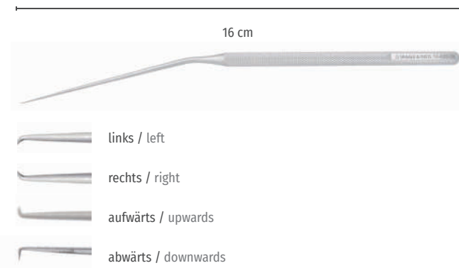
Schuknecht Mikrohäkchen, Schaft kniegebogen, 16 cm Schuknecht micro hook, angled shaft , 16 cm
