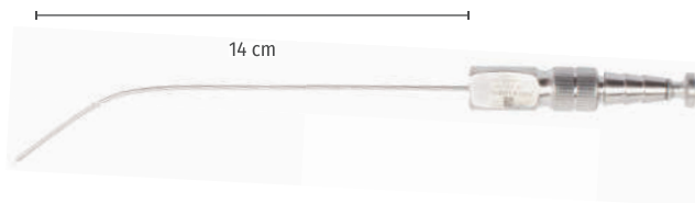
Plester Saugrohr mit Griffplatte und Unterbrecher, 14 cm Plester suction tube with suction control, 14 cm
