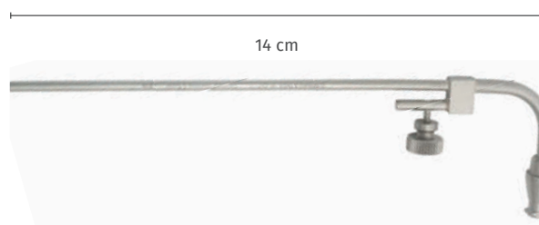
Rauchabsaugrohr für starre und spreizbare Laryngoskope Größe 3 bis 7, 14 cm Länge
