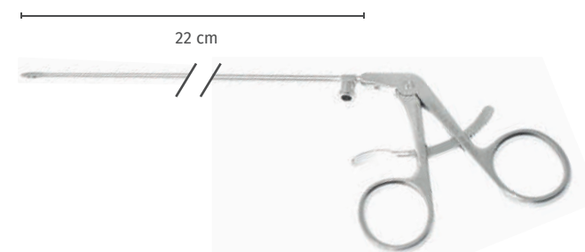
Laryngoskopie-Nadelhalter mit Spülkanal, mit Sperre, konischer Schaft (2,0 - 3,0 mm), 22 cm Laryngeal needle-holder with irrigation channel, with ratchet, conical shaft (2.0 - 3.0 mm), 22 cm 50-650-23
