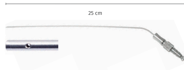
Saugrohr mit Unterbrecher, kniegebogen, seitlich distale Öffnung, 25 cm Suction tube with interruptor, angled, distal side opening, 25 cm
