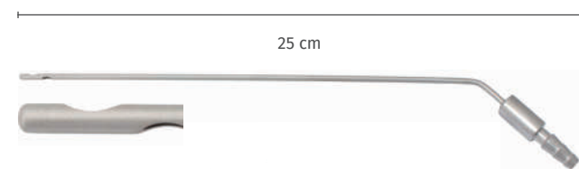
Saugrohr mit Unterbrecher, Spitze geschlossen, zwei seitliche Öffnungen 3,0 mm, 25 cm Suction tube with interruptor, tip closed, two side openings 3.0 mm, 25 cm
