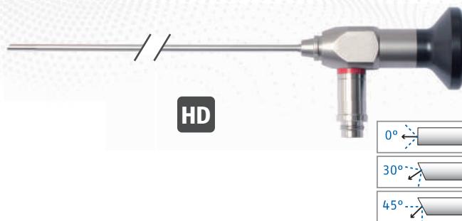
Sinuskop, HD, starr, autoklavierbar, AD 2,7 mm, 14,1 cm Sinuscope, HD, rigid, autoclavable, OD 2.7 mm, 14.1 cm
