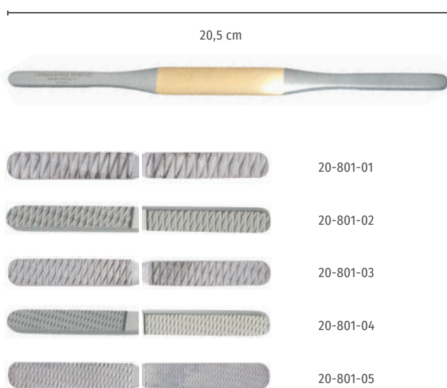
Fomon Nasenraspel, Hartmetall, doppelseitig, besonders flach, 20,5 cm Fomon nasal rasp, tungsten carbide, double ended, very flat, 20.5 cm
