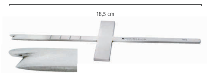
Cottle Osteotom mit Führungsdorn, gerade, 5 mm, 18,5 cm Cottle osteotome with single guard, straight, 5 mm, 18.5 cm
