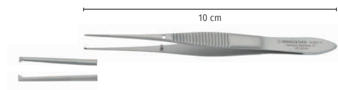
Graefe Pinzette, chirurgisch, 1:2 Zähne, gerade, 0,7 mm, 10 cm Graefe dressing forceps, 1:2 teeth, straight, 0.7 mm, 10 cm
