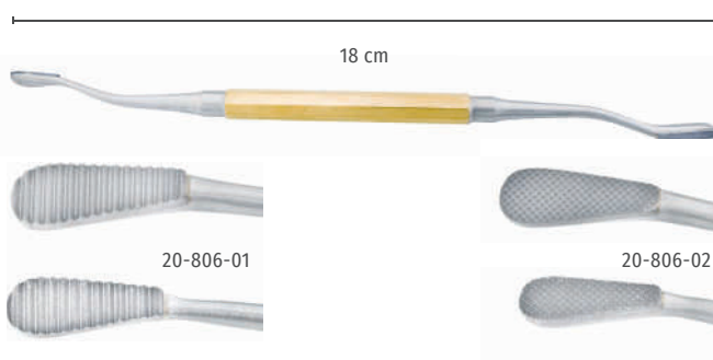
Miller Nasenraspel, Hartmetall, doppelseitig, 18 cm Miller nasal rasp, tungsten carbide, double ended, 18 cm
