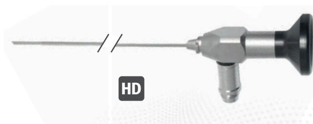
Sinuskop HD, starr, autoklavierbar, AD 4,0 mm, 17,5 cm Sinuscope, HD, rigid, autoclavable, OD 4.0 mm, 17.5 cm
